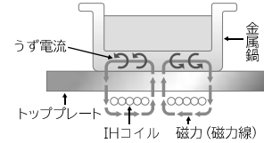
IH加熱の原理(イメージ図)
