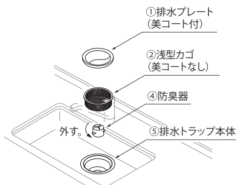
JT シンク
