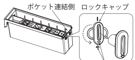
[▲] マークを合わせて取り外す
