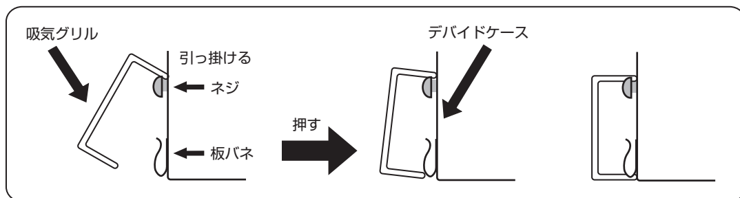
右側方から見た図
