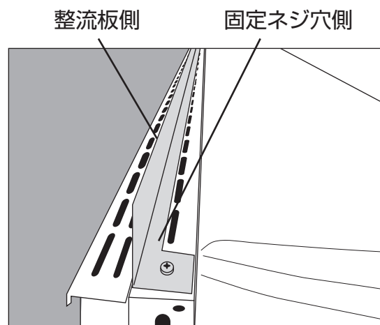
取付状態
