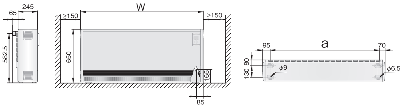
床固定位置 単位 : mm
