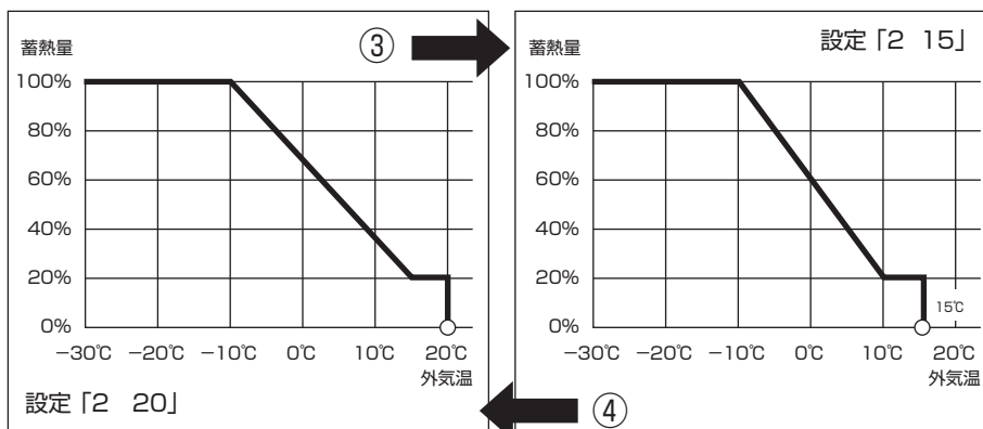
図3: 20℃で蓄熱開始
