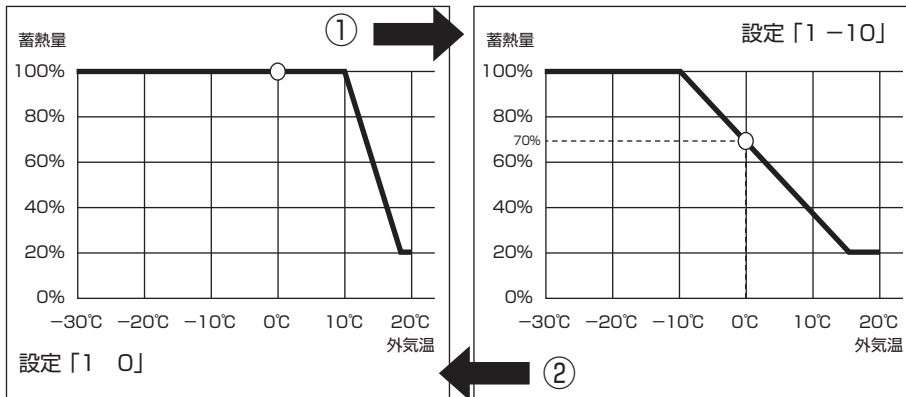
図1: 0℃で100%蓄熱
