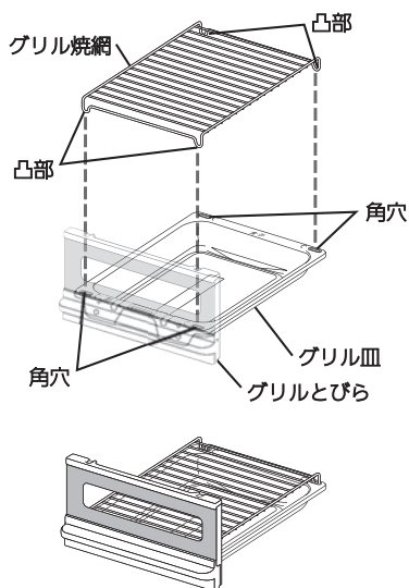
取り付け状態
