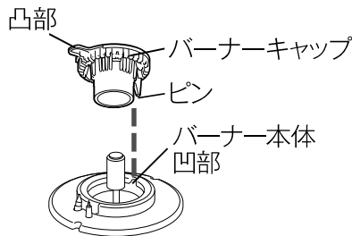
図は左／右コンロの場合
