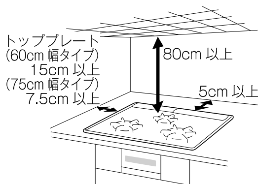
（可燃性の壁の場合）
