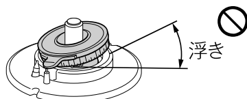
バーナーキャップの浮き
